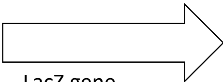
LacZ gene
