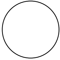
S-gal
